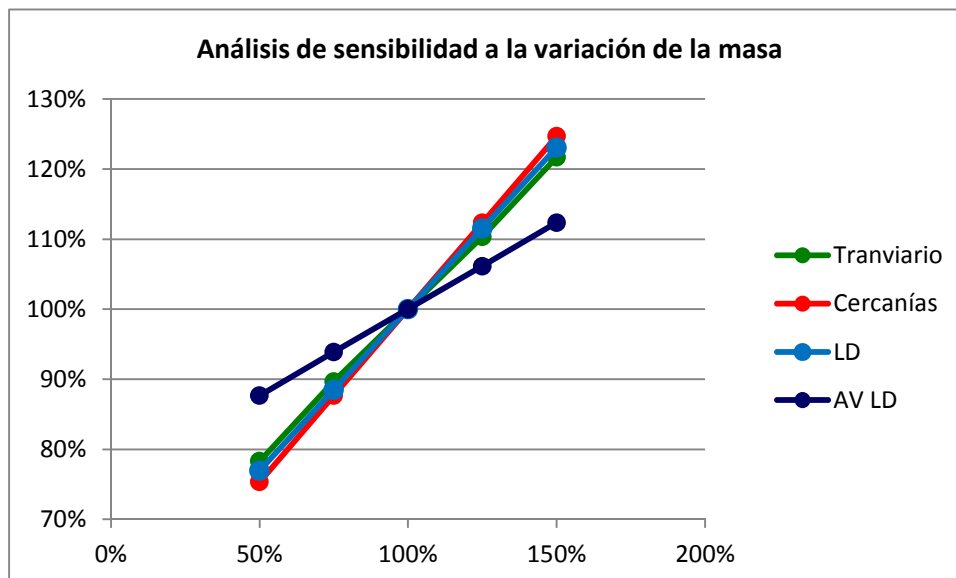
Figura 36. Sensibilidad a la variación de la masa
