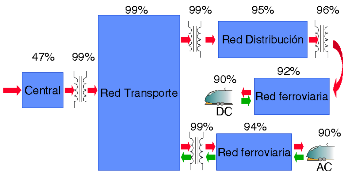
Figura 19. Eficiencia energética del ferrocarril electrificado
