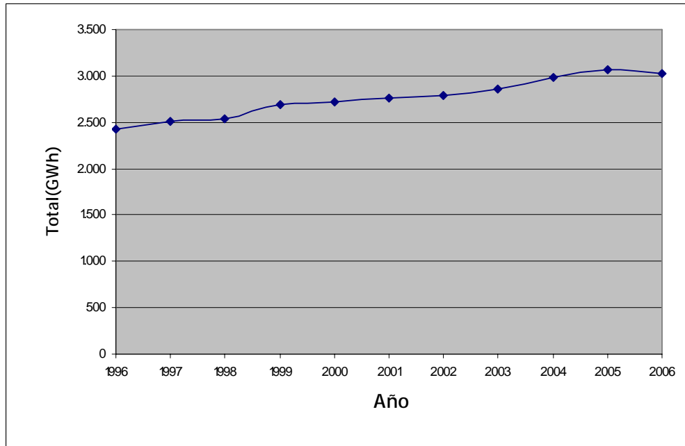
Figura 2. Consumo de energía del ferrocarril según datos de Ministerio de Fomento
